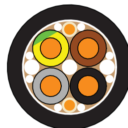
Fig. 7 Flygt HCR cable
